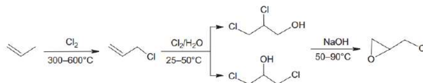
Figura 34 Proceso industrial para la obtención de la epiclorohidrina a partir del propeno
