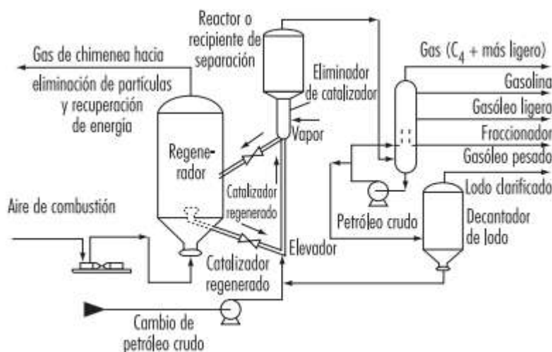
Figura 19 Proceso craqueo catalítico (35)
