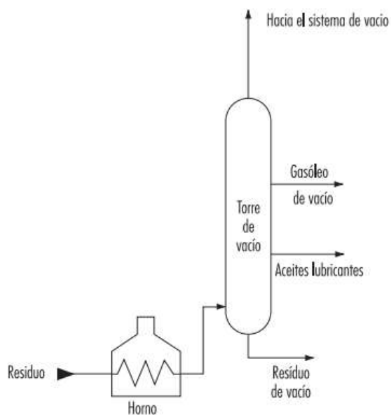
Figura 18 Proceso de destilación al vacío (35)
