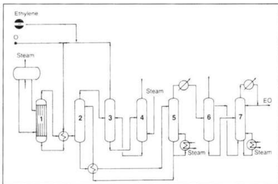
Figura 20 Proceso industrial para la obtención del óxido de etileno (1) reactor, (2) depurador, (3,4) eliminación de CO 2 , (5) decapado, (6,7) fraccionadores. (36)
