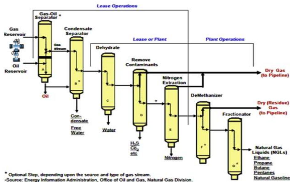
Figura 14 Diagrama general del proceso de producción de gas natural
