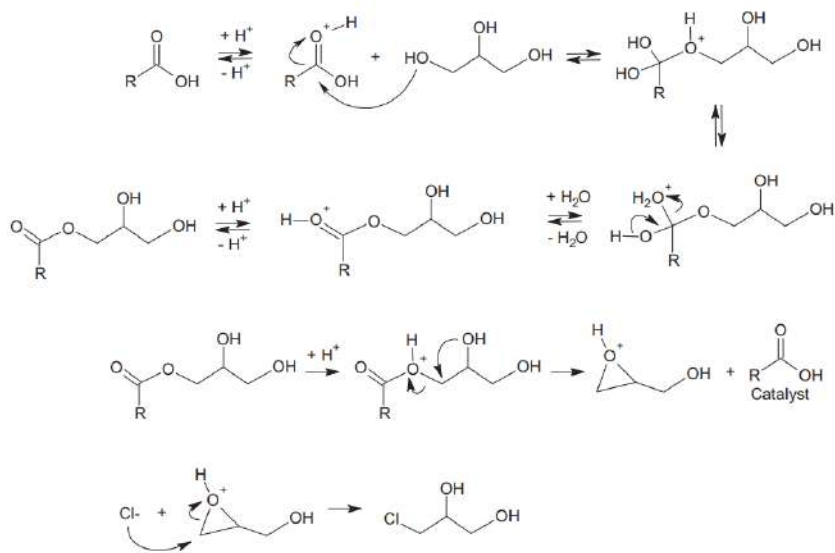
Figura 35 Mecanismo de reacción para la obtención de glicerol Clorohidrina (38)
