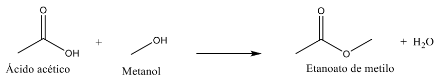
Figura 56 Síntesis de Ésteres
