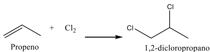
Figura 58 Halogenación de alquenos
