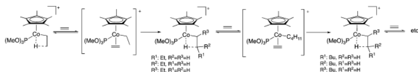
Figura 5 Mecanismo de polimerización del etileno (15)
