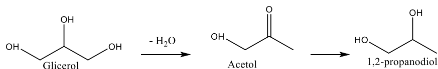
Figura 37 Obtención del 1,2-propanodiol
