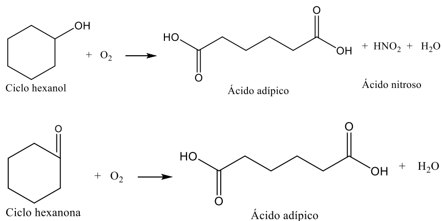
Figura 46 Oxidación del ciclo hexanol y ciclo hexanona
