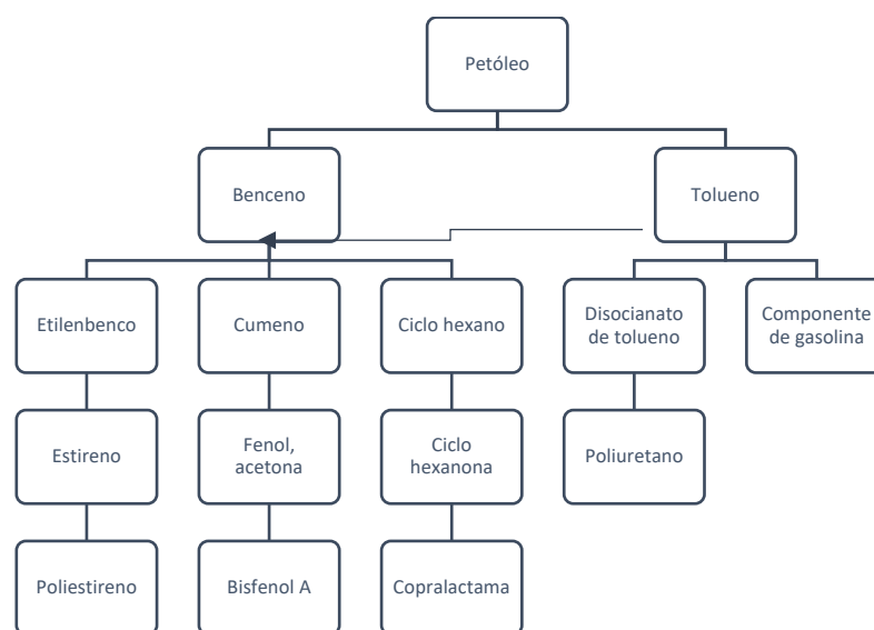
Figura 1. Algunos derivados a partir del petróleo.
