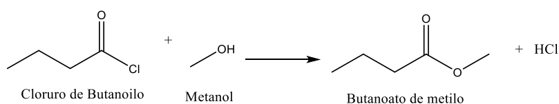
Figura 61 Síntesis de ésteres mediante coluros ácidos
