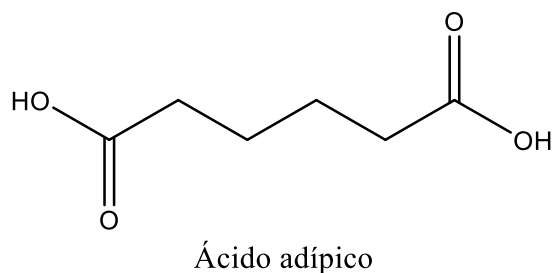
Figura 45 Estructura ácido adípico
