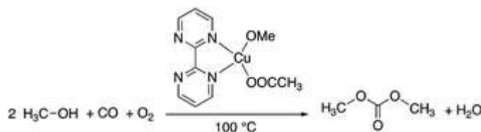
Figura 8 Carbonilación oxidativa del metanol en dimetilcarbonato (26)
