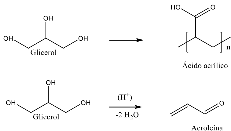
Figura 38 Obtención del ácido acrílico y acroleína
