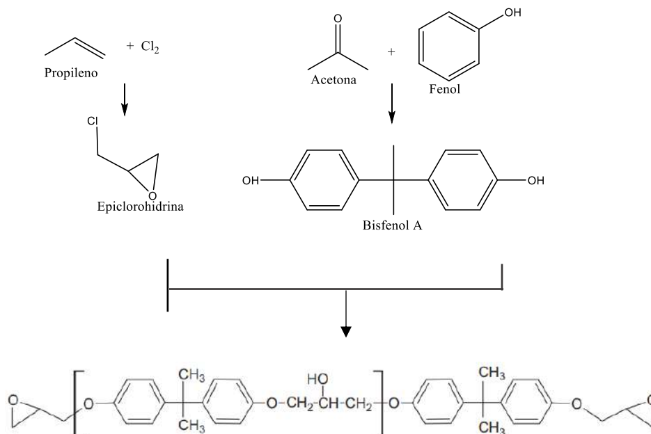
Figura 36 Obtención de resinas epoxi
