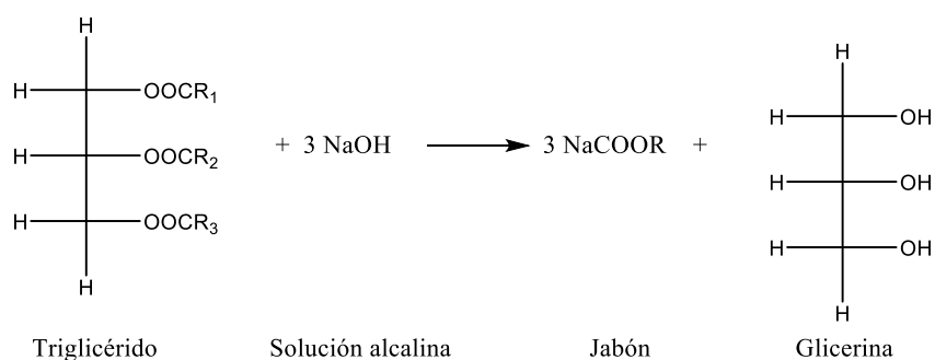
Figura 63 Reacción de Saponificación
