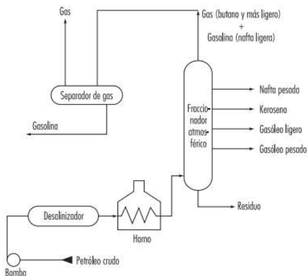
Figura 17 Proceso de destilación atmosférica (35)
