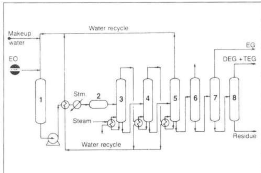
Figura 21 Esquema industrial de producción del etilenglicol (1) tanque de alimentación, (2) reactor, (3,4,5) evaporadores de múltiples etapas, #4 opera a menor presión que el #3, mientras que el #5 opera bajo vacío, evaporado el agua se recicla al tanque de alimentación, (6) separador de extremos ligeros, (7,8) columnas de destilación al vacío. (36)
