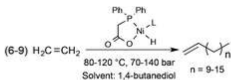
Figura 10 Oligomerización del etileno (28)
