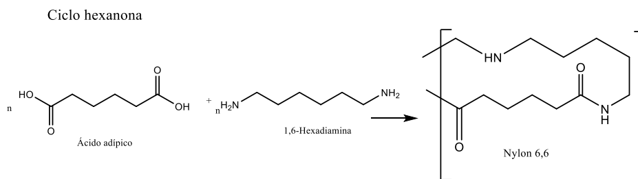
Figura 47 Síntesis del Nylon 6,6
