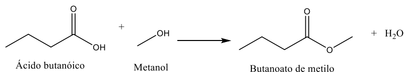
Figura 60 Reacción de esterificación
