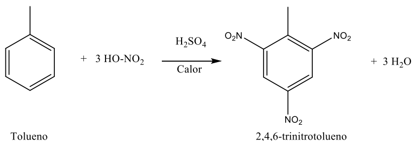
Figura 64 Síntesis de TNT
