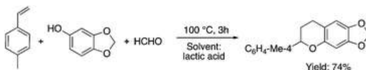
Figura 9 Reacción del ácido láctico (27)
