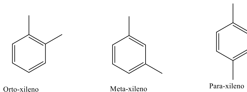
Figura 41 Xilenos posición orto meta y para
