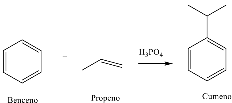
Figura 43 Síntesis del Cumeno
