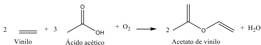
Figura 62 Síntesis del acetato de vinilo
