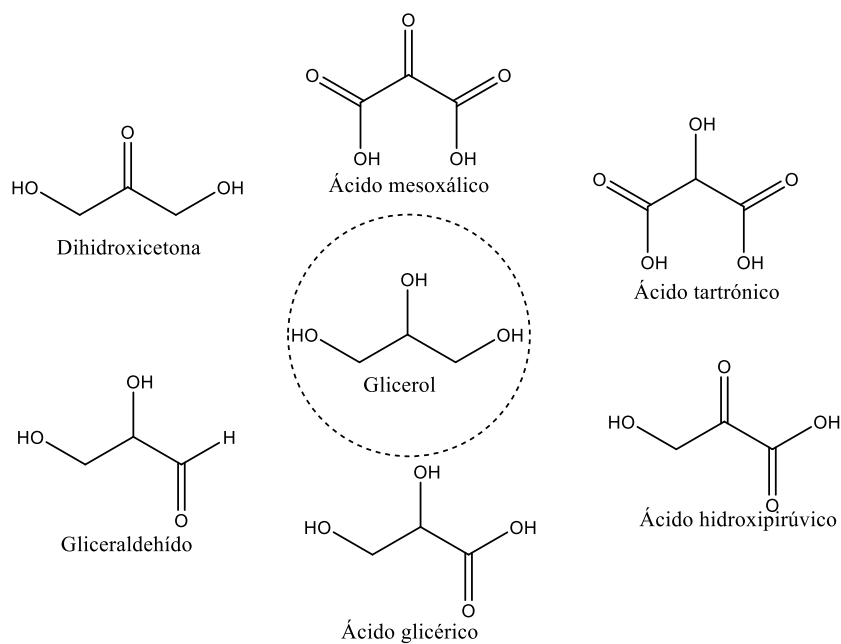
Figura 39 Productos obtenidos a partir de la oxidación del glicerol.
