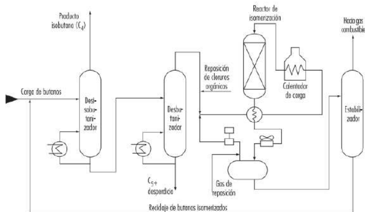
Figura 40 Isomerización del Butano.
