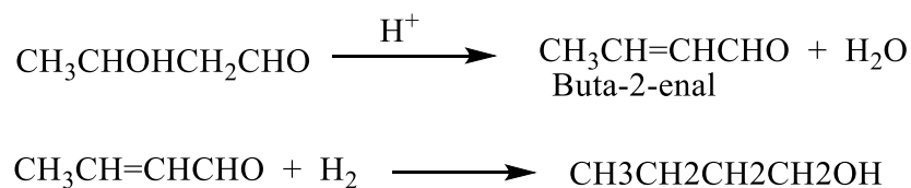
Figura 27 Obtención del butanol a partir del 3-hidroxibutanal
